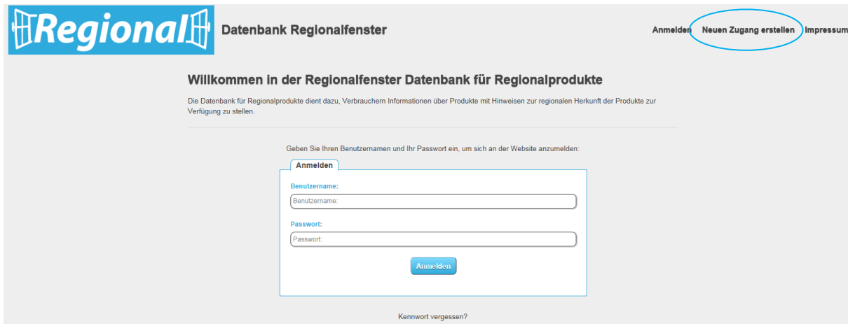
Abbildung 1: Datenbank-Regionalfenster Startseite
